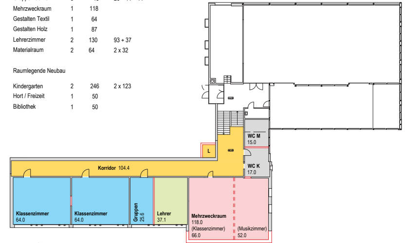
2. Obergeschoss
