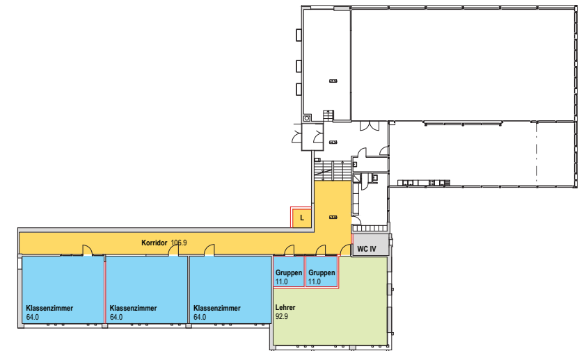
1. Obergeschoss
