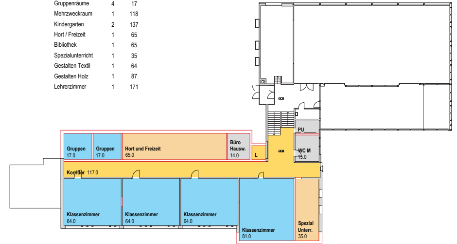
2. Obergeschoss
